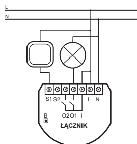
Rys.1 Schemat elektryczny podłączenia Łącznika Fibaro.
